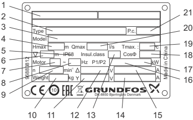
Obr. 13 Typový štítek
