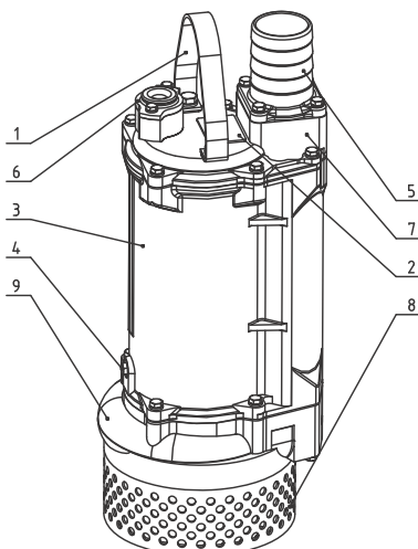
Obr. 11 Čerpadlo DWK
