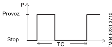
Obr. 8 Provoz S3
