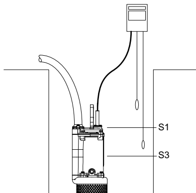
Obr. 7 Provozní hladiny DWK
