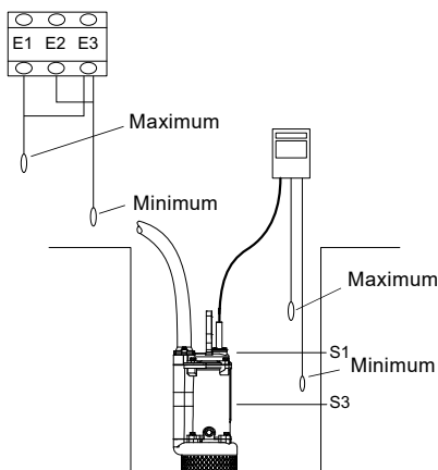
Obr. 14 Řídicí jednotky čerpadel
