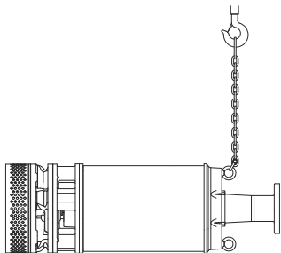
Obr. 1 Zdvžení výrobku do vzpřímené polohy, krok 1
