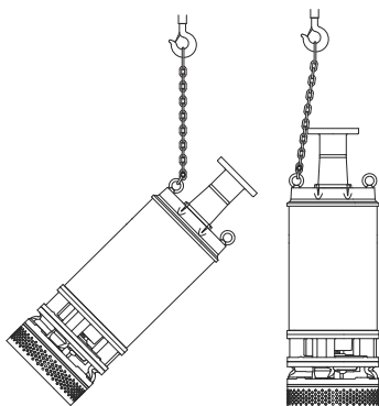
Obr. 2 Zdvžení výrobku do vzpřímené polohy, krok 2
