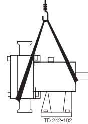
Čerpadlo bez příslušenství
